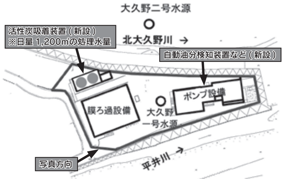
大久野浄水所施設平面図
