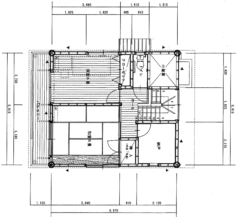
2階平面図 1/50
