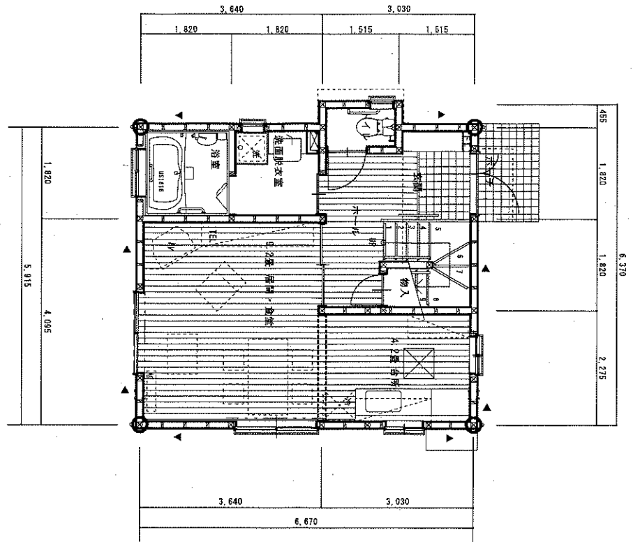
1階平面図 1/50
