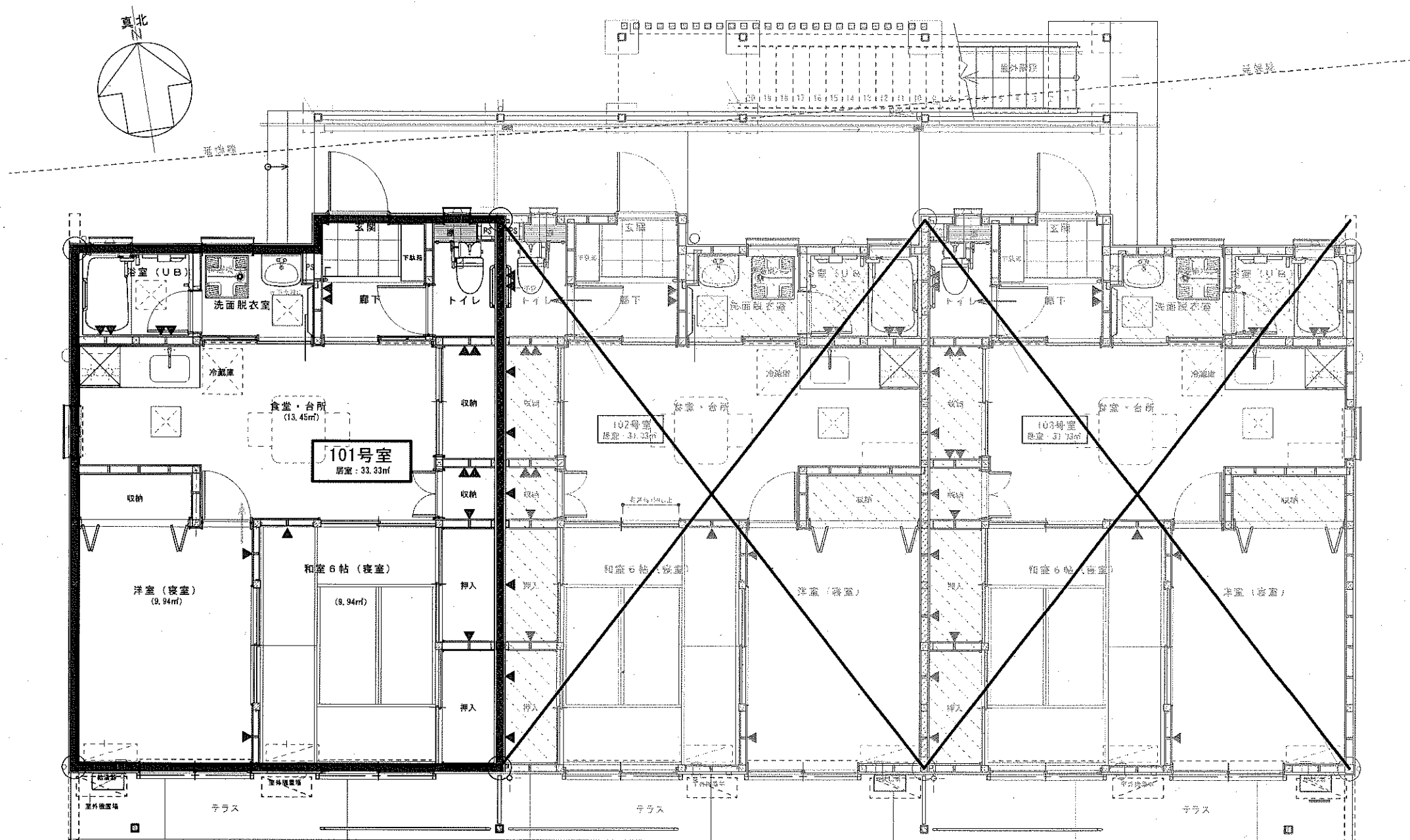
諏訪下住宅C棟 1階平面図
