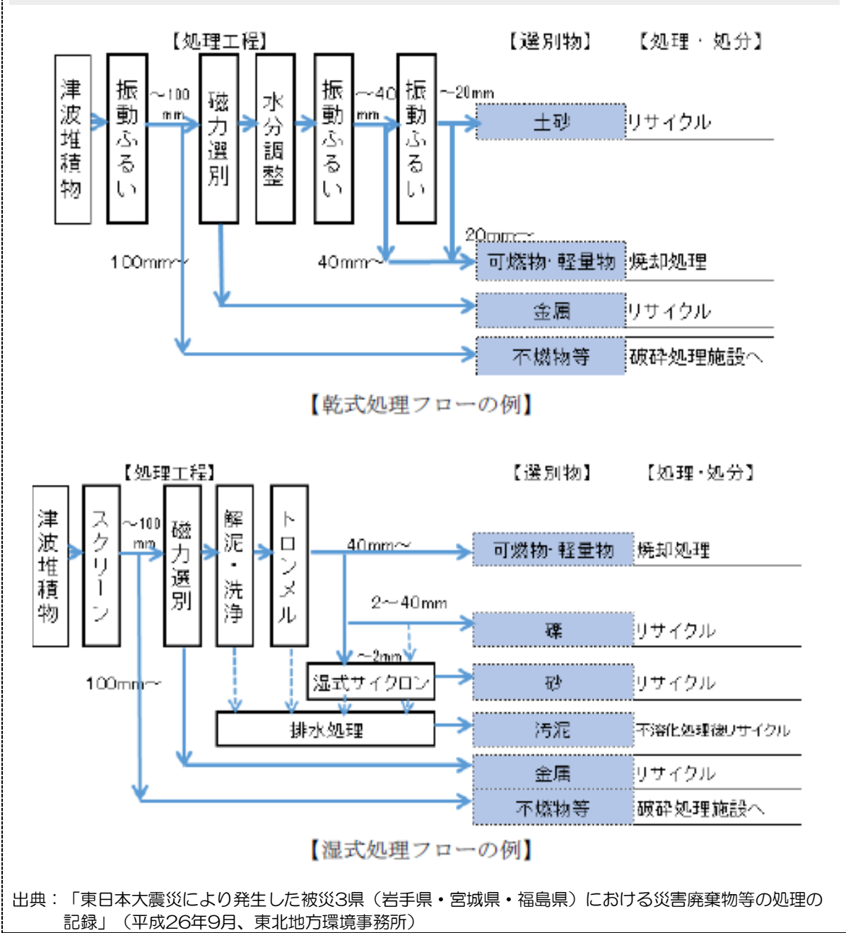
図表6-12 津波堆積物の処理（例）
